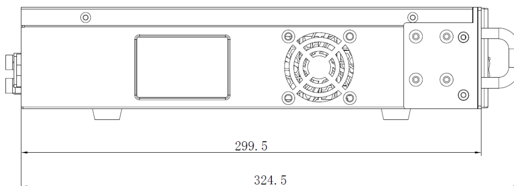
侧面尺寸图
