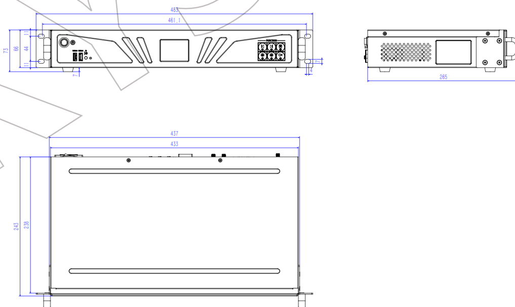
设备尺寸图
