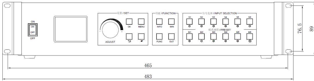
前面板尺寸图
